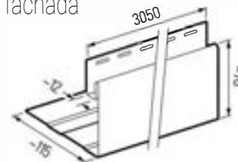
SV 17 Tapajuntas pequeño de fachada
