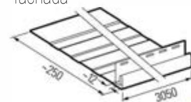
SV(P) 19 Tapajuntas grande de fachada
