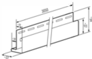
SV(P) 16.5 Drip edge
