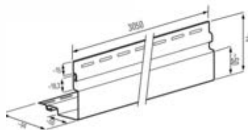
SV 17 Tapajuntas pequeño de fachada
